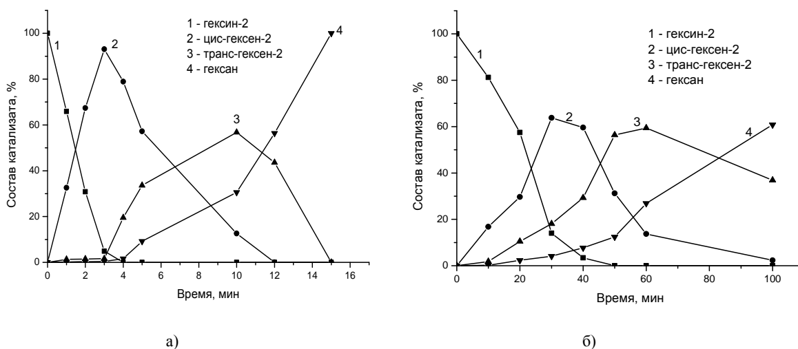
Рисунок 1 – Изменение состава катализата во времени при гидрировании гексина-2 на 1%Pd-Ni(3:1)-ПЭГ/ZnO (а) и 1%Pd-Ag(3:1)-ПЭГ/ZnO (б) катализаторах
