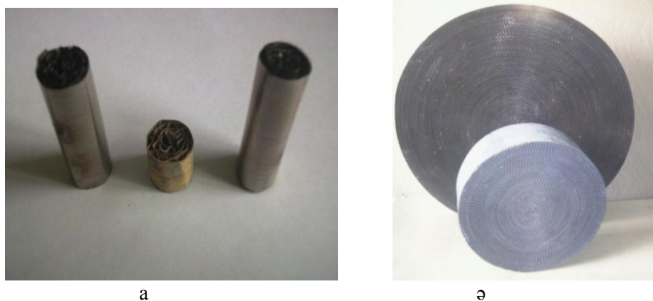
Сурет 1 - Металды блокты тасымалдағыштағы катализаторлар: а- зертханалық үлгі, ә- автотранспорттың табиғи газдарын сынауға арналған үлгілер
