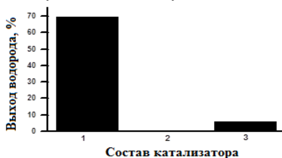
Рисунок 4 - Влияние состава активной фазы катализатора на выход водорода при C 3 -C 4 УВ:O 2 :N 2 :Ar=0,95:1:3,76:0,95, T=550 0 С, V=3150 ч -1
