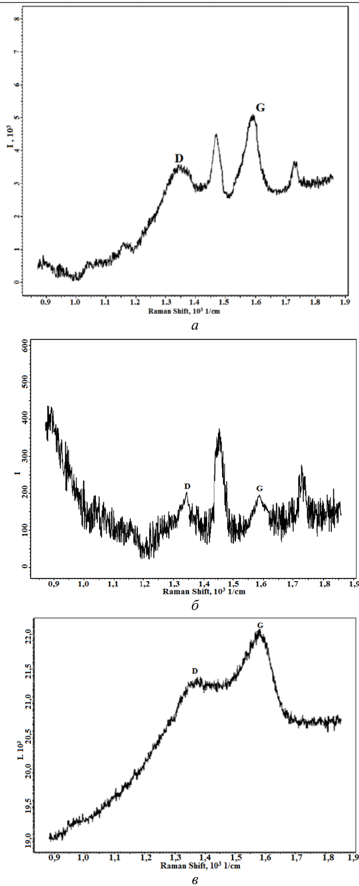
5-сурет – Көміртектің Раман- спектрлері: а – бірінші аймақ, б – екінші аймақ, в – үшінші аймақ
