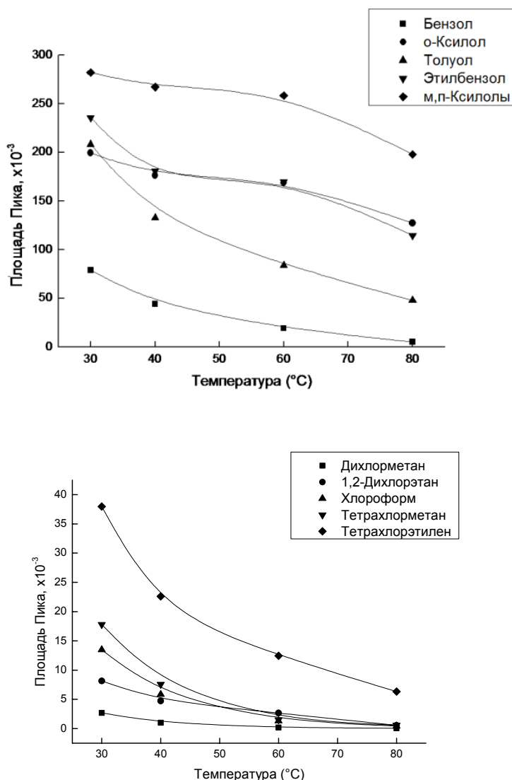
Рисунок 2 – Зависимость площади пиков ЛОС (БТЭЖ и ХОС) от температуры экстракции
